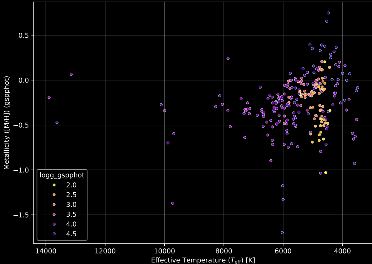
APOGEE DR17 Field: [ORIONOB1AB-D] Stellar Population Parameters (n= 262)
